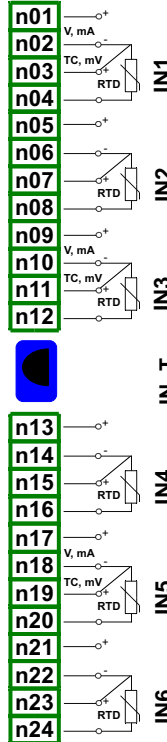
QFUN6 6 universal inputs
