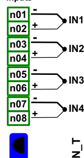
TC8 8 thermocouple inputs
