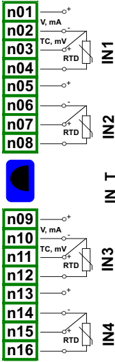
EFUN4 4 universal inputs
