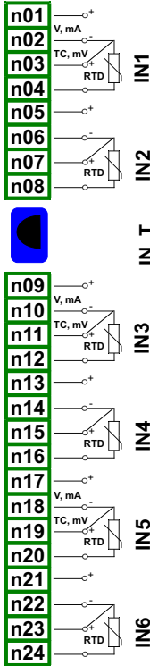
EFUN6 6 universal inputs
