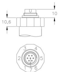
Binder serie 723 7-pin (IP 67)
